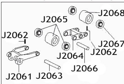
Wahacz z łącznikiem zespolonym
