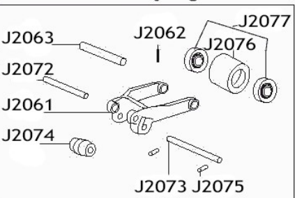
Wahacz z rolką singiel
