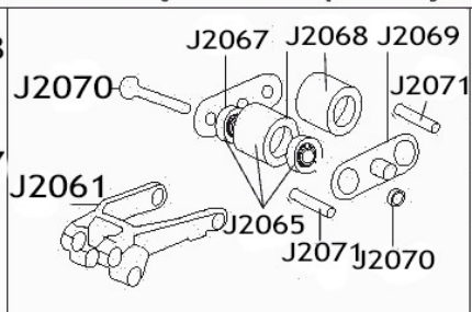
Wahacz z łącznikiem trzpieniowym
